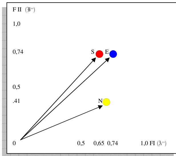
Abbildung 2: Vektorielle Orte der AST-SEN-Skalen
